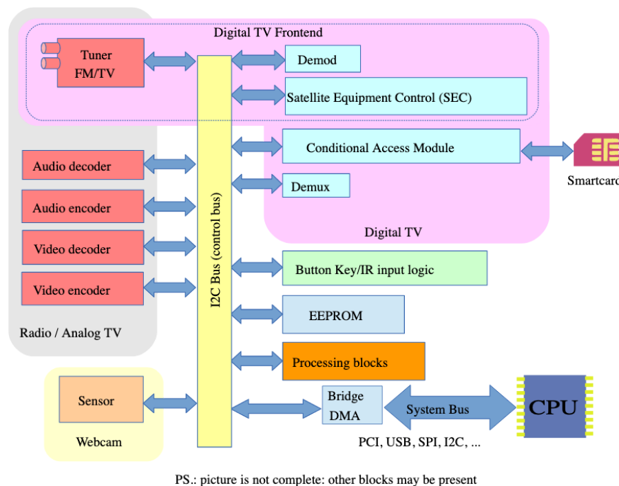
Figura 2.2. Comunicación entre dispositivos de multimedia [25].
