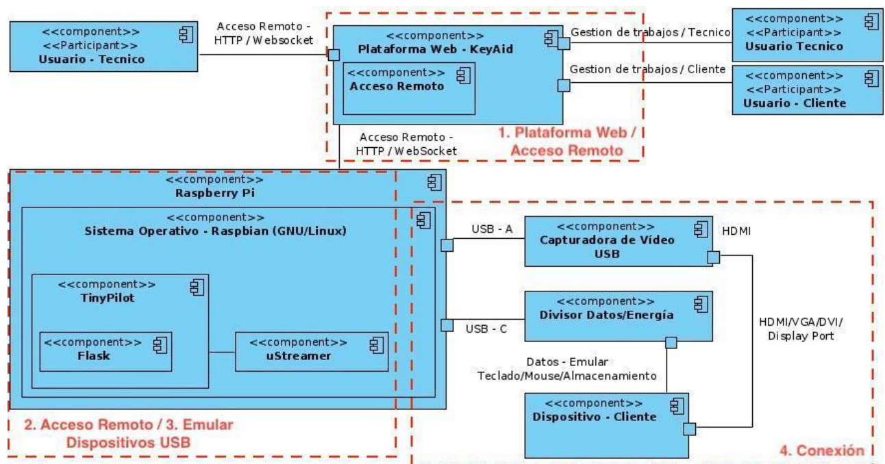
Figura 3.1. Modelo de componentes de “KeyAid”
