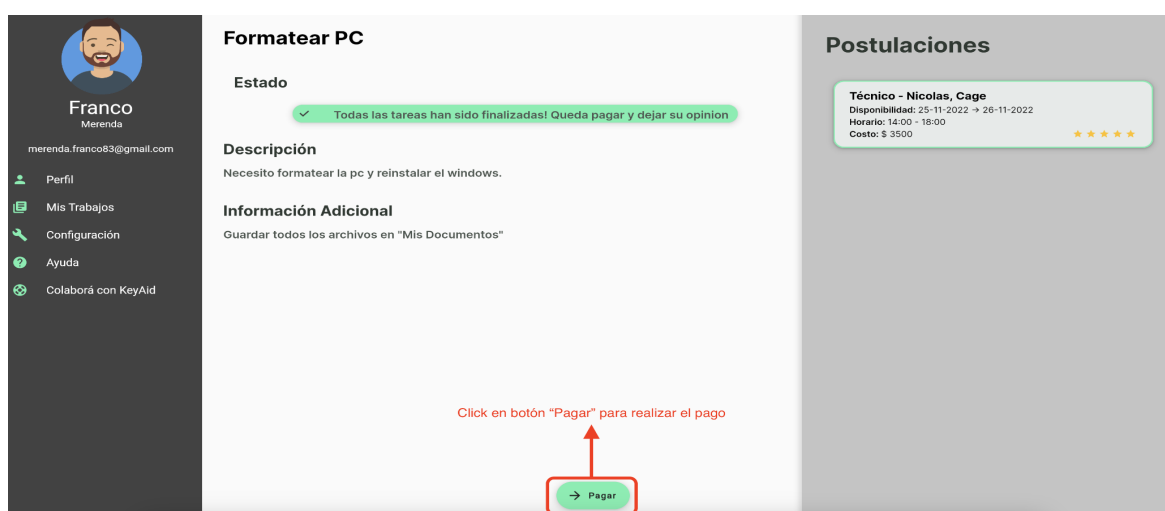
Figura A2.13 - Pantalla de trabajo - Botón para realizar el pago
